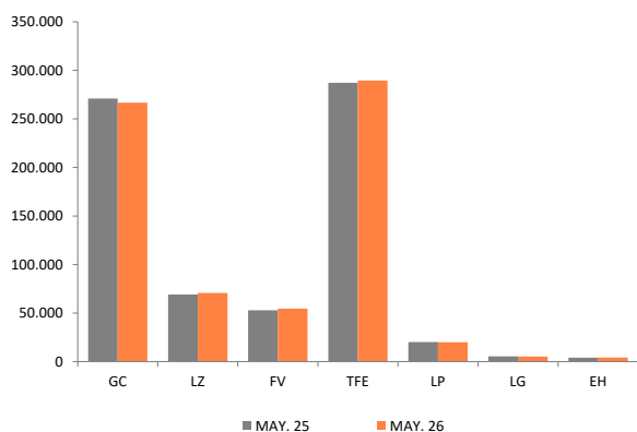
ENERGÍA ELÉCTRICA DISPONIBLE SEGÚN ISLAS (Mwh) MAY. 25-26
