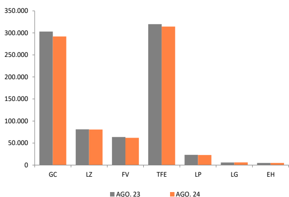
ENERGÍA ELÉCTRICA DISPONIBLE SEGÚN ISLAS (Mwh) AGO. 23-24
