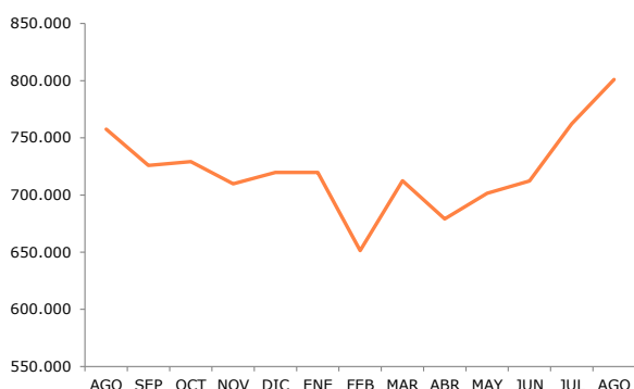
ENERGÍA ELÉCTRICA DISPONIBLE. CANARIAS (Mwh) AGO. 22-23
