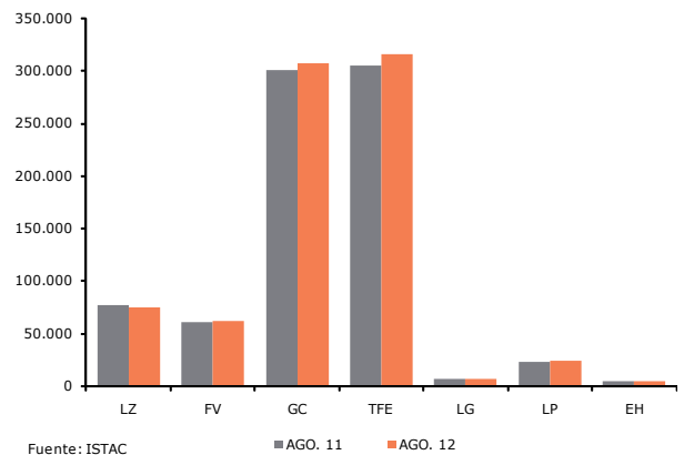
ENERGÍA ELÉCTRICA DISPONIBLE POR ISLAS (Mwh) AGO. 11-12
