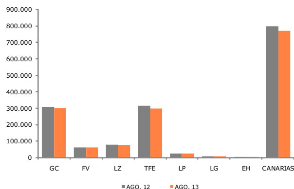
ENERGÍA ELÉCTRICA DISPONIBLE SEGÚN ISLAS (Mwh) AGO.12-13
