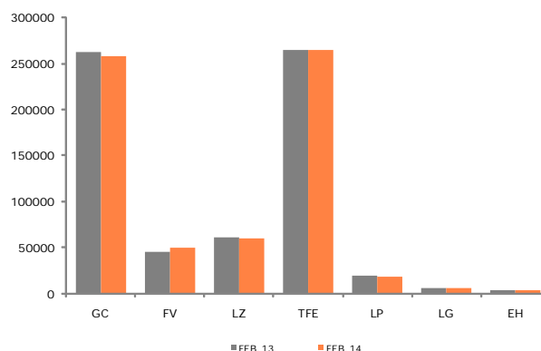
ENERGÍA ELÉCTRICA DISPONIBLE SEGÚN ISLAS (Mwh) FEB 13-14
