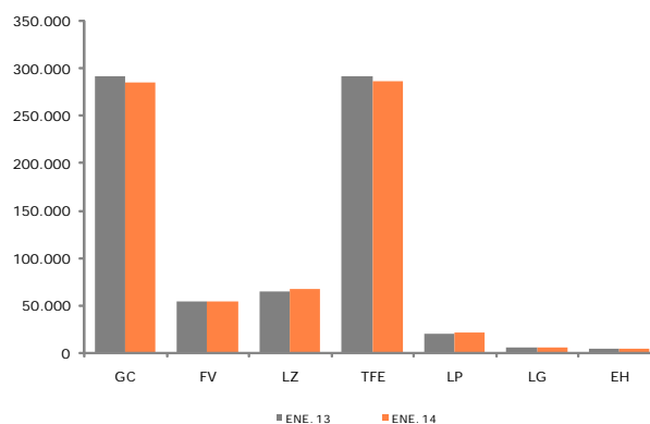
ENERGÍA ELÉCTRICA DISPONIBLE SEGÚN ISLAS (Mwh) ENE 13-14
