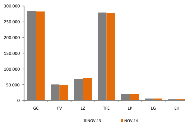
ENERGÍA ELÉCTRICA DISPONIBLE SEGÚN ISLAS (Mwh) NOV 13-14
