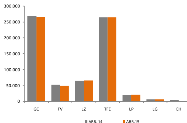
ENERGÍA ELÉCTRICA DISPONIBLE SEGÚN ISLAS (Mwh) MAY 14-15
