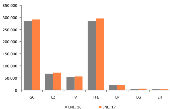
ENERGÍA ELÉCTRICA DISPONIBLE SEGÚN ISLAS (Mwh) ENE. 16-17
