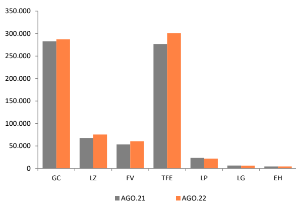
ENERGÍA ELÉCTRICA DISPONIBLE SEGÚN ISLAS (Mwh) AGO. 21-22
