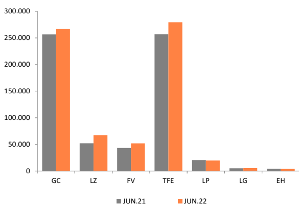
ENERGÍA ELÉCTRICA DISPONIBLE SEGÚN ISLAS (Mwh) JUN. 21-22
