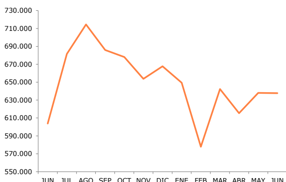
ENERGÍA ELÉCTRICA DISPONIBLE. CANARIAS (Mwh) JUN. 20-21
