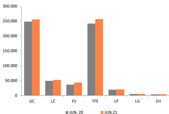
ENERGÍA ELÉCTRICA DISPONIBLE SEGÚN ISLAS (Mwh) JUN. 20-21
