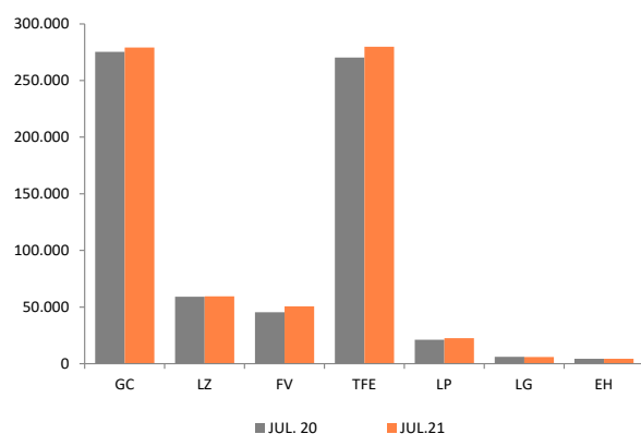
ENERGÍA ELÉCTRICA DISPONIBLE SEGÚN ISLAS (Mwh) JUL. 20-21
